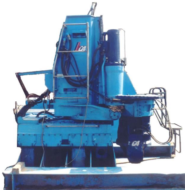
Máy ép cọc tĩnh
