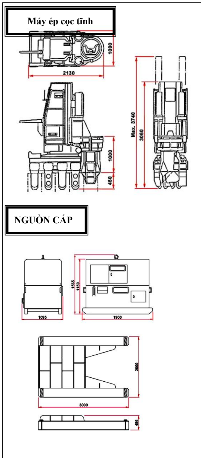
Máy ép cọc tĩnh
